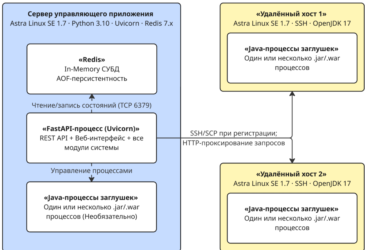
Рисунок 4 – Диаграмма развёртывания
